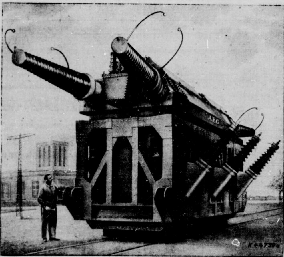
Werkphoto: AEG.
