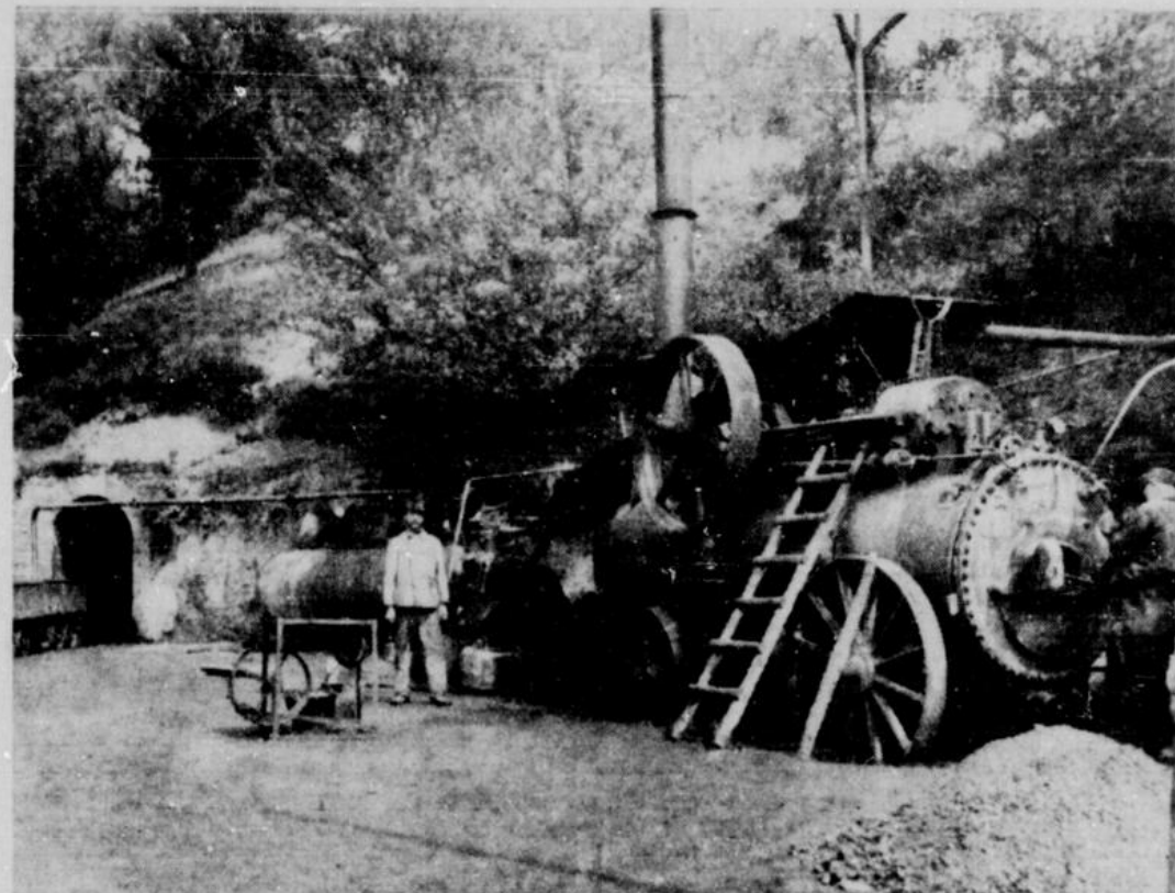
Eine Freiluft-Bergwerks-Maschinenanlage
