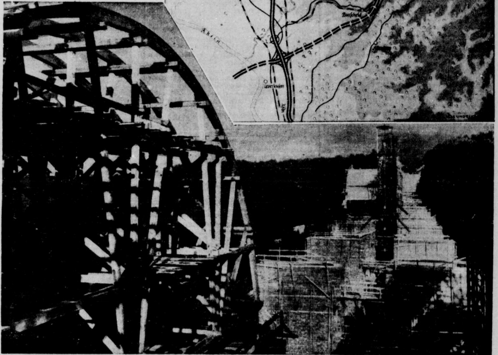
Brücke am Einsiedelstein bei der Heintjesmühle im Eschbachtal. 350 m lang, 36 m hoch. 7 Gewölbe mit Grauwackeverkleidung und Basaltavabögen.
