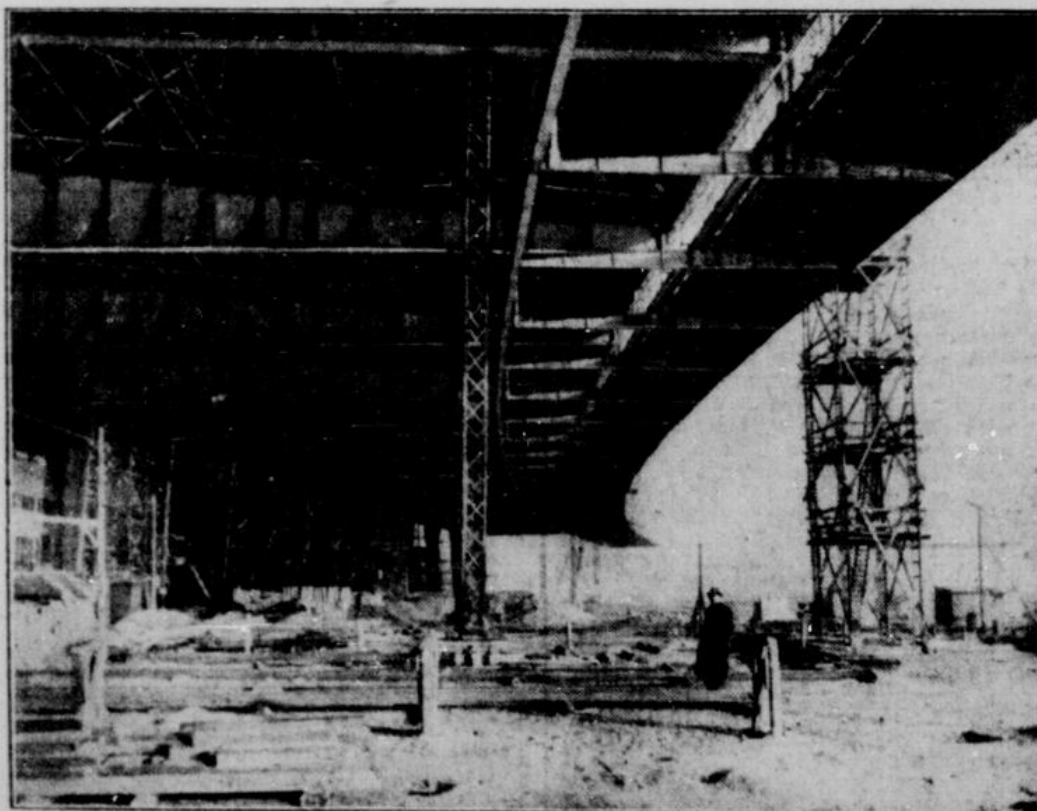
Der neue Zentralflughafen Berlin-Tempelhof (Flugbahnsteig und Abfertigungsgebäude).
