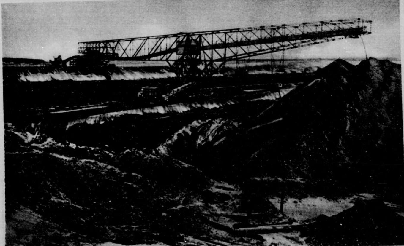
Abraum-Förderbrücke der Grube Golpa. Stundenleistung 2150 cbm, Stützenweite 180 bis 200 m, Auslegerlänge 120 m
