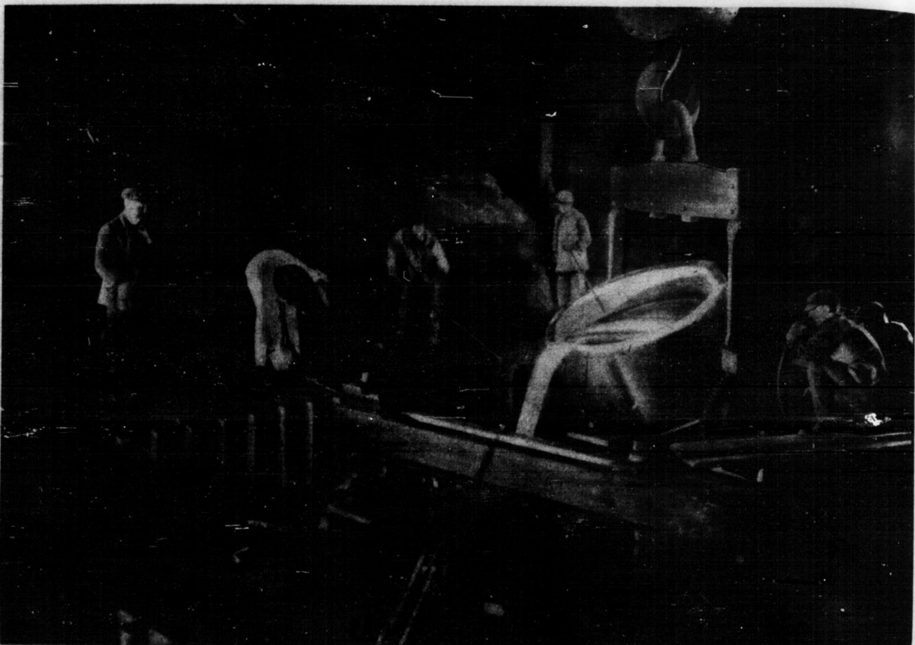
Guß eines schweren Gasmaschinenzylinders aus einer 20000-kg-Pfanne Die schwere Verankerung der Form ist gut zu sehen. Die Form ist in der Stiefgrube verankert. Anton W. Tiedt
