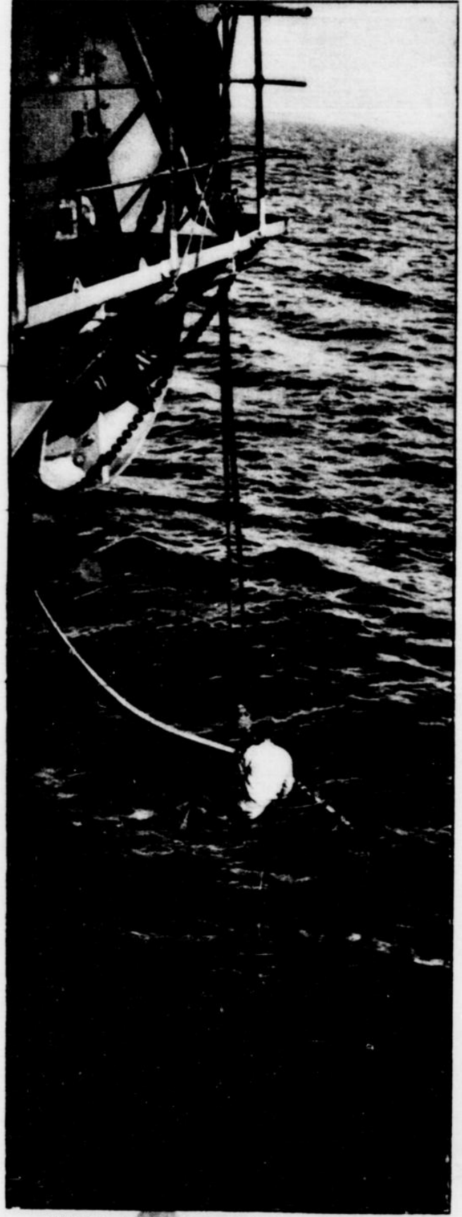
Abtropfen des Kabels vor Anfertigung eines Splisses (Verbindung zweier Kabelenden)
