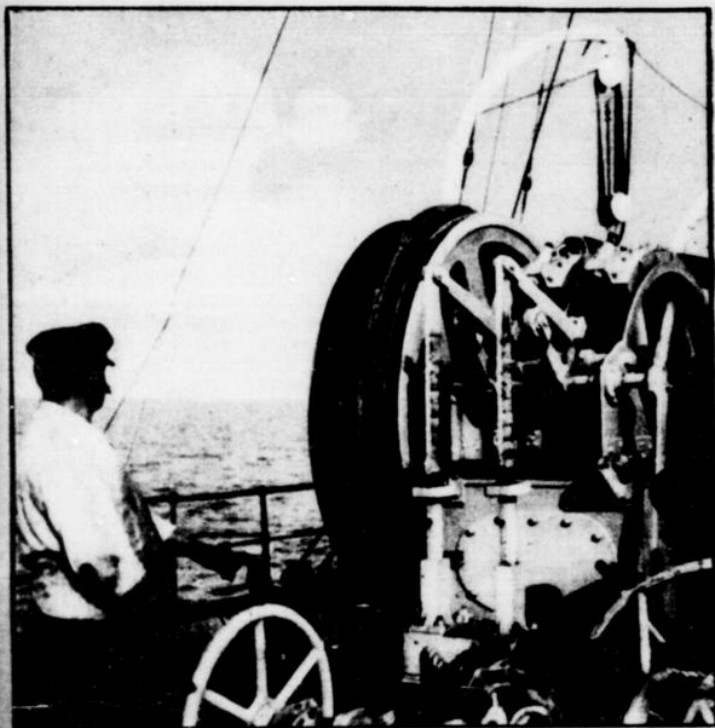
Kabelanlegemaschine mit Bremsvorrichtung
