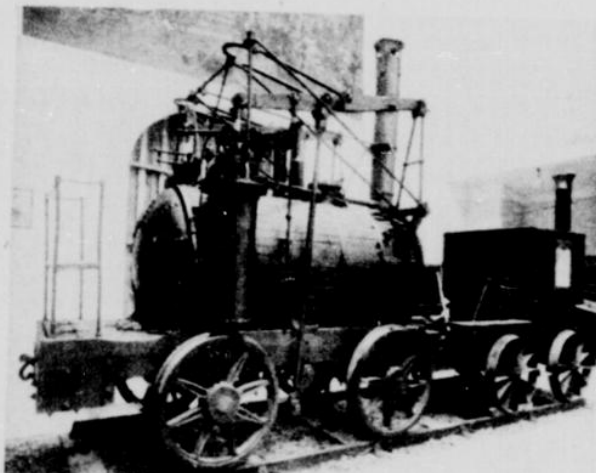
Nachbildung der ersten Lokomotive, die zur Beförderung von Kohlezügen diente (1813 in England erbaut, Original im Kensington-Museum in London.) Fahrtgeschwindigkeit mit 10 beladenen Kohlenwagen 8—10 km in der Stunde
