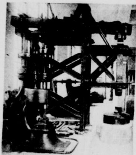
Das Modell des Dampfhammers „Alter Fritz“ von Krupp, im Vordergrund: Der älteste Dampf- hammer der Linke-Hofmann-Werke, Breslau
