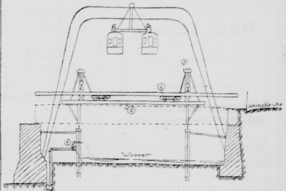
2. Die Aufstellung der Fundamentträger für den Neubau des Schwebebahnhs Döppersberg.
