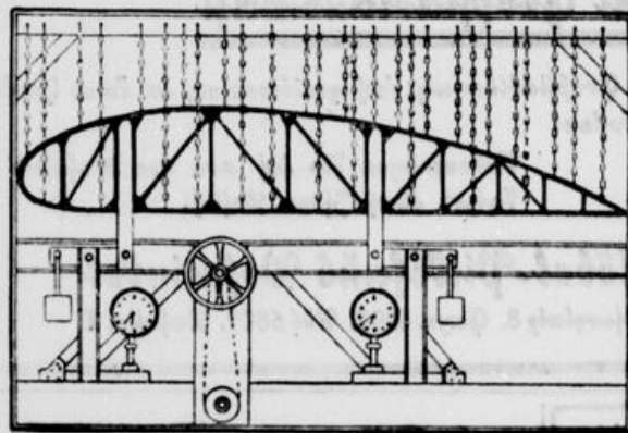
Festigkeitsprüfung von Flugzeugrippen
