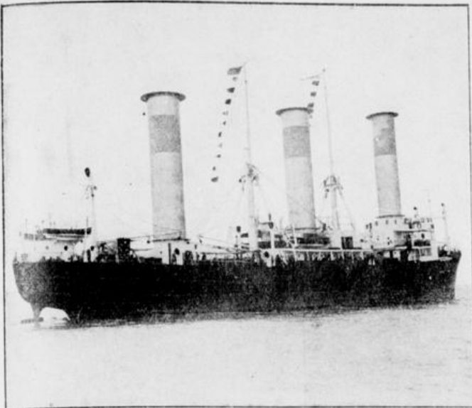
Das im Auftrage der Marineleitung erbaute Motor-Rotor-Schiff „Barbara“ trat am 30. Juli von Bremerhaven aus seine letzte Erprobungs- und zugleich Übergabefahrt nach Hamburg an. Photothek
