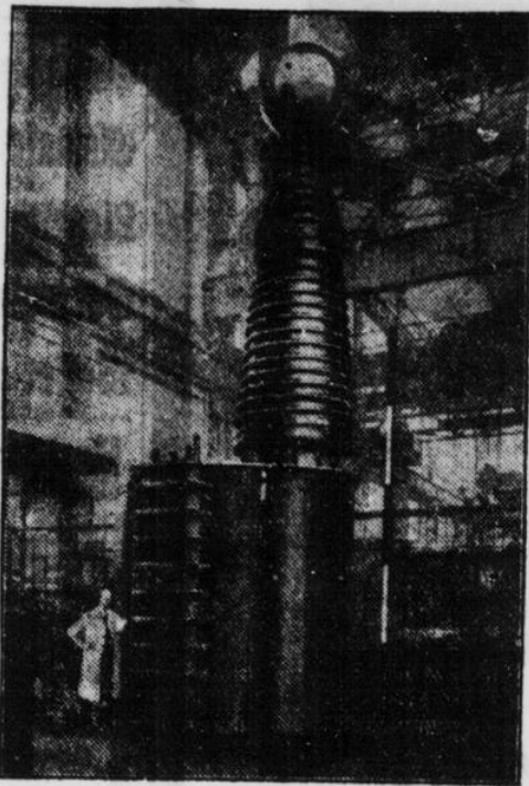
Ein Prüftransformator für eine Million Volt. Das Gerät ist über 8 Meter hoch und wiegt über 31 Tonnen.
