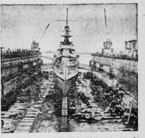
Das 50 000 Tonnen-Dock in Singapur versenkt Bei einem Angriff der japanischen Heeresluftwaffe wurde das große britische Schwimmdock von 50 000 Tonnen Tragfähigkeit getroffen und versenkt.
