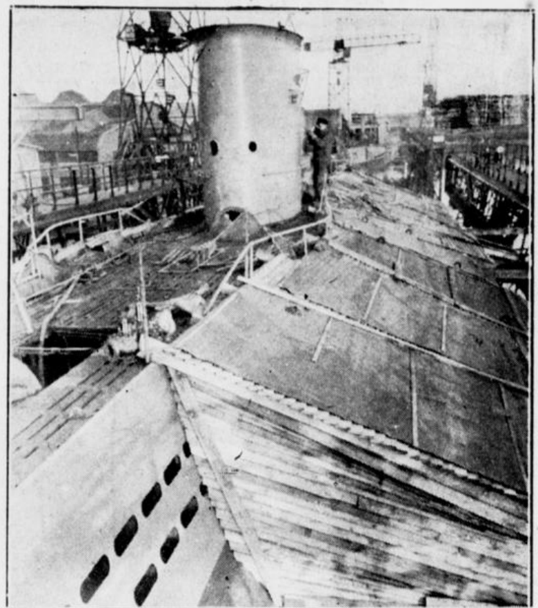
U-Boot im Trockenock. Die Arbeit geht Tag und Nacht vor sich. Um die notwendigen Arbeiten trotz der Verdunkelung auch nachts durchführen zu können, hat man über die Arbeitsstellen Holzverschaltungen gebaut, die keinen Lichtschimmer durchlassen.
