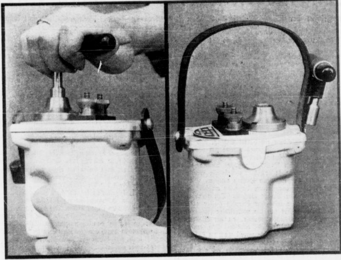
Neukonstruktion eines elektrischen Minenzünders für Bergwerke und Steinbrüche (links im Gebrauch, rechts tragfertig).
