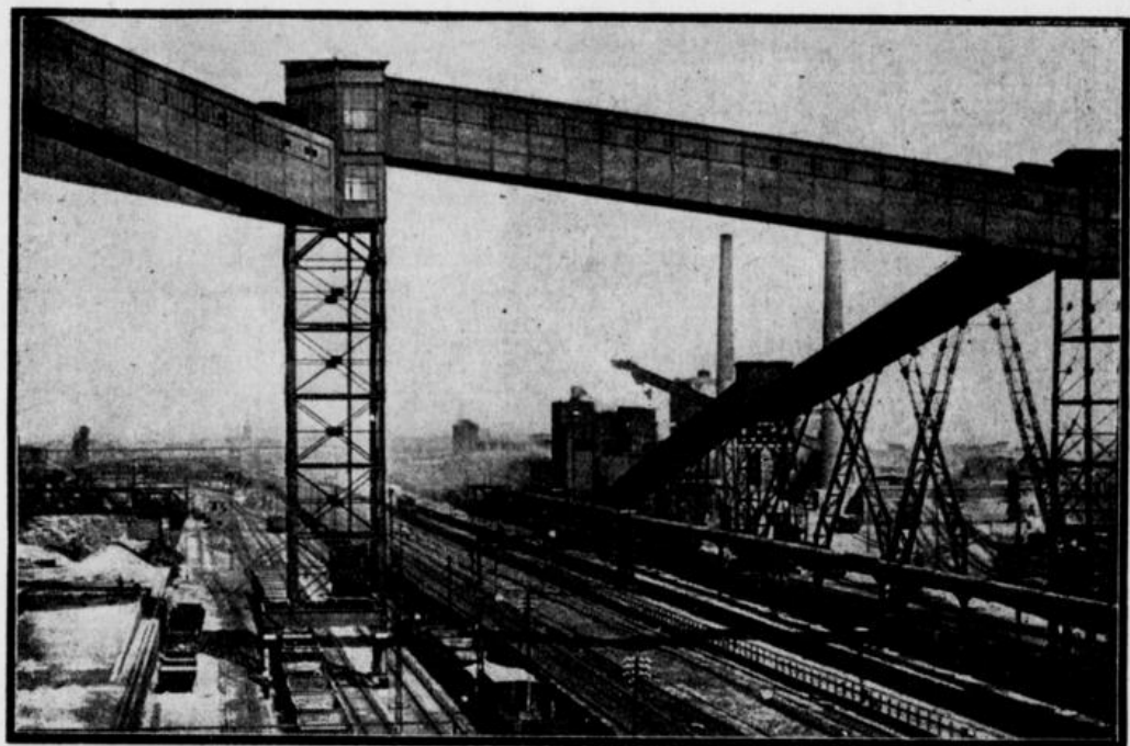
Die Brücke zwischen den Hochöfen und Kokerei Alma
