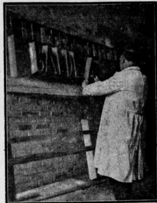
Im Brennofen werden zu brennenden Waren untergebracht. Der weiße Raum wird mit zwei Mauern verschlossen.
