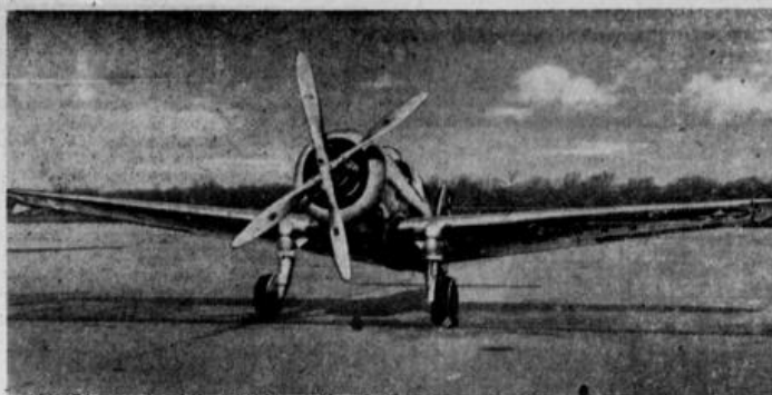
Die Luftfahrtabteilung des amerikanischen Kriegsministeriums hat erfolgreiche Versuche mit einem neuen Propeller durchgeführt, der eigentlich aus zwei Propellern besteht, die sich in entgegengesetzter Richtung bewegen. Unser Bild zeigt das Versuchsfeld mit den entgegengesetzt laufenden Luftschrauben. Weltbild (K)
