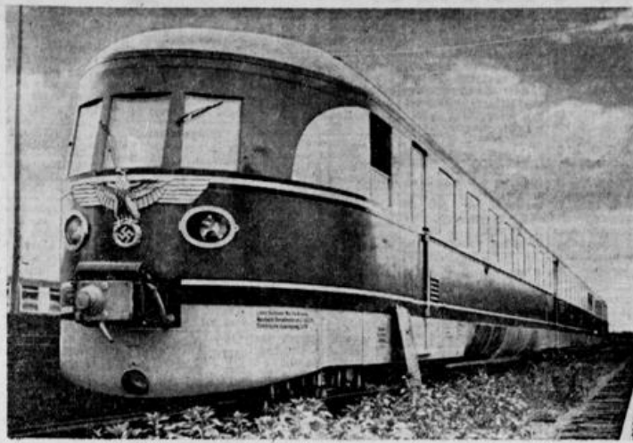
Der neue Schnelltriebwagen der Reichsbahn, der auf der Strecke Berlin-Köln in Dienst gestellt wird. Der Wagen, der mit zwei Diesel-Elektromotoren zu je 600 PS ausgestattet ist, erreicht eine Geschwindigkeit von 160 std/km. Weltbild (K)
