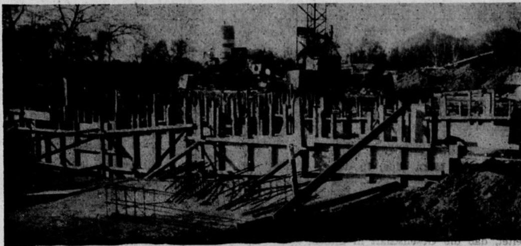
Die Arbeiten zum Neubau des Inseleiswimmbades gehen zügig voran. Mit dem Gießen der Fundamente für das Eingangsgebäude ist bereits begonnen worden. HVZ-Fotos: Günter Groote
