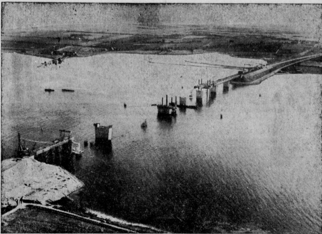
Die 960 Meter lange Brücke über den Fehmarnsund, die im Zuge der Vogelfluglinie errichtet wird, wächst immer mehr nach Norden. Das Luftbild gibt einen interessanten Ueberblick über die im Bau befindliche Brücke. Mit Hilfe von Hubseilen werden die sieben stählernen Nebenträgerwerke montiert. Im Sommer 1963 soll die Vogelfluglinie in Betrieb genommen werden.
