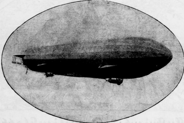
Das Zeppelin-Luftschiff Sachsen, das, als 17. auf der Friedrichshafener Werft erbaut, der „Delag“ gehört und in Leipzig stationiert wurde, ist 140 Meter lang, hat 14,8 Meter Durchmesser, fast rund 20.000 Kubikmeter und ist mit einer Maschine für 20 Fahrgäste versehen. Die funktentelegraphische Anlage gestattet, von Bord des Luftkreuzers bis auf 500 Kilometer Zeichen zu geben und solche bis 1000 Kilometer her zu empfangen. Die Maschinen entwickeln 435 Pferdestärken und mit zwei Motoren eine Geschwindigkeit von 16,5 Sekundenmetern. Mit drei Motoren legt das Passagierflugschiff etwa 20 Sekundenmeter, also 72 Kilometer in der Stunde, zurück.
