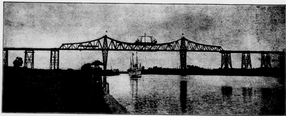
Die neue Eisenbahnhochbrücke über den Kaiser-Wilhelm-Kanal. Am 1. Oktober soll die neue Eisenbahnhochbrücke über den Kaiser-Wilhelm-Kanal bei Mendeburg in Betrieb genommen werden. Während jetzt die beiden Eisenbahnstrecken Hamburg-Altenburg und Kiel Quäsum auf zwei Drehbrücken in Mithöhe über den Kanal geleitet werden, führt die neue Hochbrücke die Bahn 33 m höher als bisher über den Kanal und erleichtert den Eisenbahn- wie den Schiffsverkehr. Die gewaltige Brücke hebt sich in der flachen Landschaft besonders auffallend ab. Sie ist etwa 500 m lang, und die Eisenbahndämme liegen 44 m über dem Wasserspiegel des Kaiser-Wilhelm-Kanals. Um die Züge von dem ebenen Boden allmählich höher zu heben, waren auf beiden Kanalseiten umfangreiche Erdarbeiten und die Erbauung großer Stützwerke erforderlich. Das vollendete Bauwerk ist ein neues Meisterstück deutscher Technik, denn an Größe nur die 60 m hohe und 300 m lange Eistalbrücke sowie die 80 m hohe und 550 m lange Gölzhofbrücke gleichkommen.
