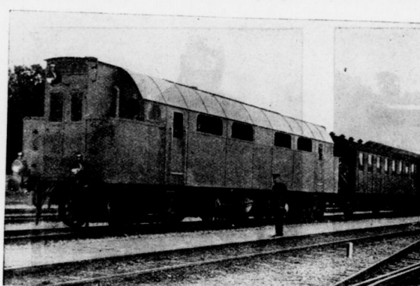
Eine Motorschlothe, die mit einem der auch in der Seefahrt be-währten Dieselmotoren versehen ist und mit gutem Erfolg Probefahrten machte.
