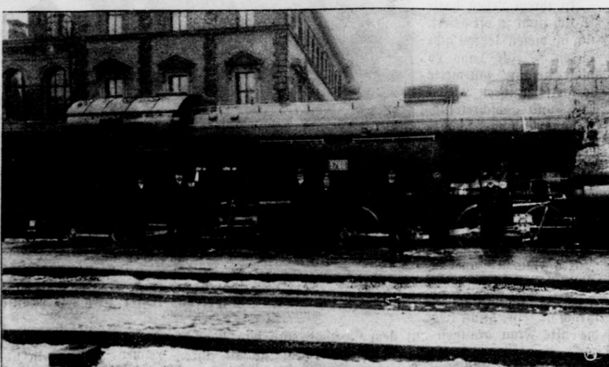
Die größte Güterzuglokomotive Europas, die wir hier zeigen, ist auf der bayerischen Eisenbahn verwendet und als Heißdampf-Tenderlokomotive System Mallet von der bekannten S. A. Maschinenfabrik in München erbaut worden. Diese Schiebelokomotive ermöglicht große Ersparnisse. Ein Bild von der Größe der Maschine geben folgende Zahlen: Länge der Lokomotive von Puffer zu Puffer gemessen 17,55 Meter, Zahl der Räderachsen 8, Gewicht 450 Zentner, Zugkraft 18250 Kilo, Betriebsdruck des Kessels 15 Atmosphären, Wasserkraft des Kessels 8350 Liter. — (Phot. Bericht Hoffmann.)
