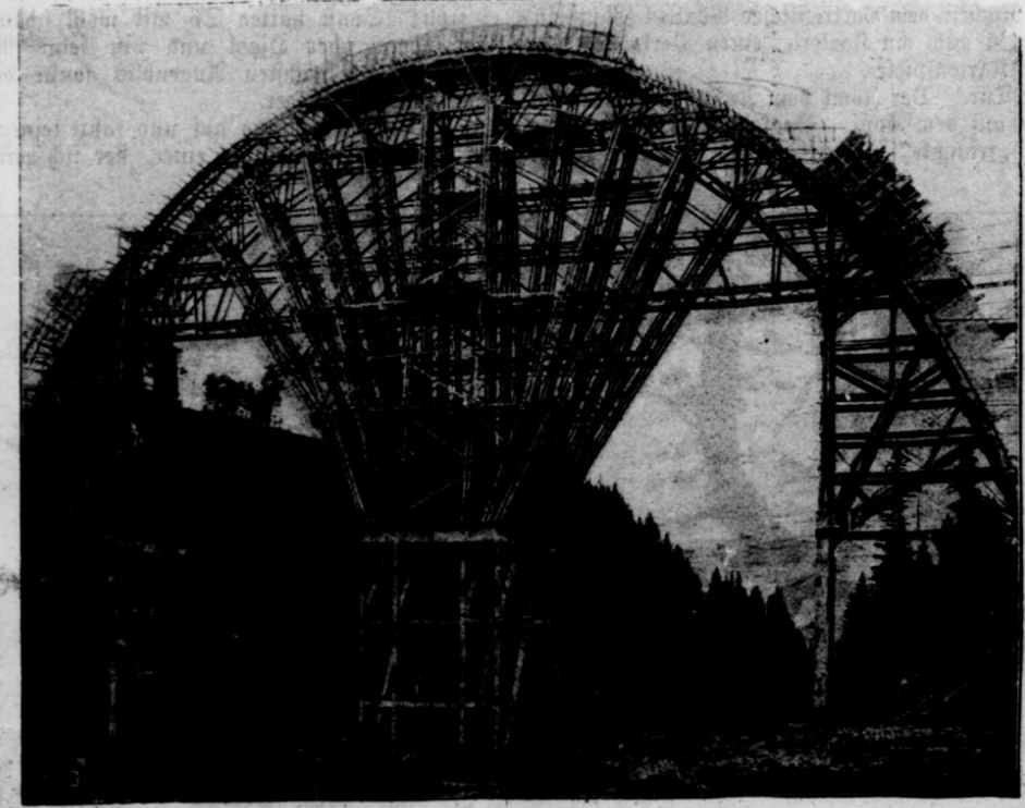
Die größte Bogenbrücke der Welt aus Eisenbeton. Der Baudukt von Langwies auf der neuen elektrischen Chur-Arosa-Bahn, der die Aescherschlucht in 70 m Höhe überbrückt, wird die größte Bogenbrücke aus Eisenbeton sein, die bisher hergestellt worden ist. Die Brücke ist 237 m lang und die Spannweite des Bogens beträgt 100 m.
