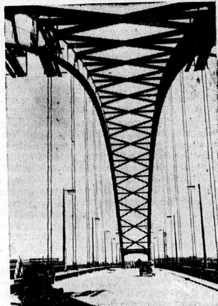
Die neue Straßenbrücke über den Rhein zwischen Duisburg und Rheinhausen wurde kürzlich feierlich dem Verkehr übergeben. Mit ihrem großen Mittelbogen, der die über 250 Meter breite Hauptstromführung überspannt, ist sie die größte stählerne Bogenbrücke in Europa. Sie ist die wichtigste Verkehrsverbindung zwischen dem Ruhrgebiet und dem Gebiet links des Niederrheins sowie den Beneluxländern.
