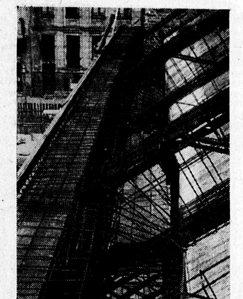
Die Stützpunkte der massiven Stahlbetonbinder an der Längswand der Halle
