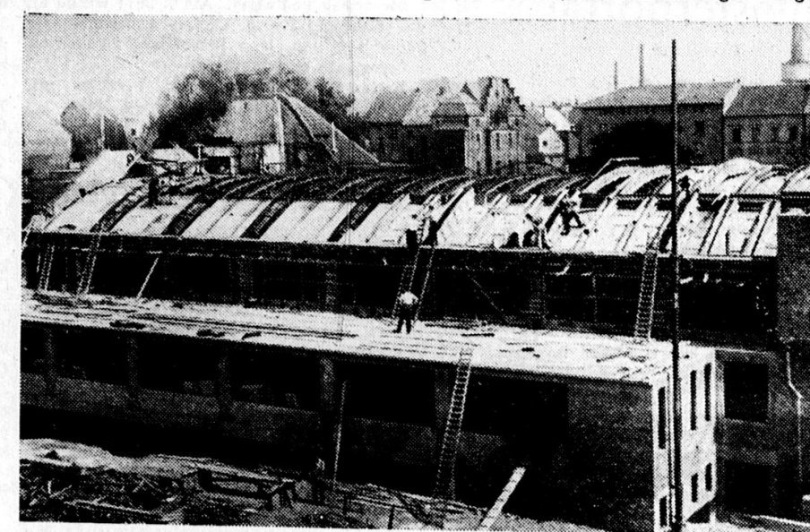
So sieht das neue Hallenbad heute aus. Eine Frage: Könnte man auf dem Dach der „Seiten-schiffe“ nicht eine Liegewiese zum Sonnenbaden einrichten? (natürlich mit Abschuß gegen die Schwannstraße hin und mit Baumkulissee).
