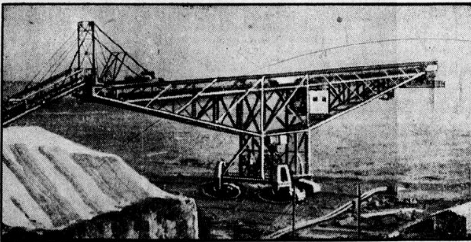
Auf einer rheinischen Braunkohlengrube kam die erste von der I.G. vollständig elektrisch ausgerüstete Abraumförderbrücke mit Raupenfahrwerk in Betrieb. Die drei das Bauwerk tragenden Ruppen haben die ungewöhnlichen Abmessungen von 9 Meter Länge, 3 Meter Höhe und 2 Meter Breite.
