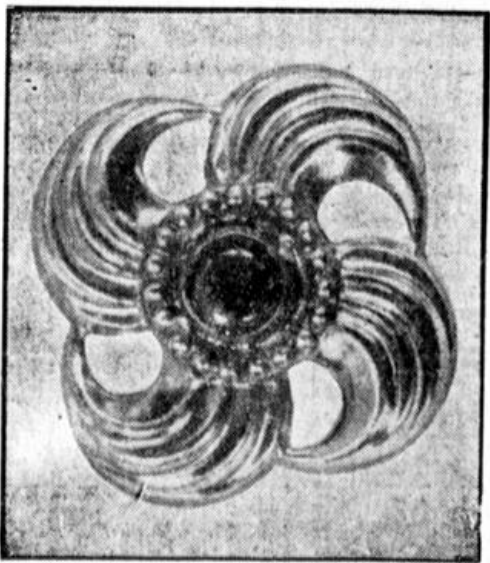
Weltbild (M).
