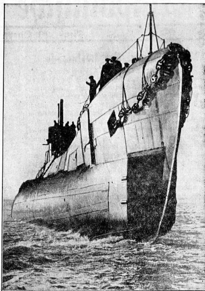
Der englische Unterseekreuzer „Severn“ nach dem Stapellauf. Man beachte die feihte Wulstform, die durch die Taufs bedingt wird.
