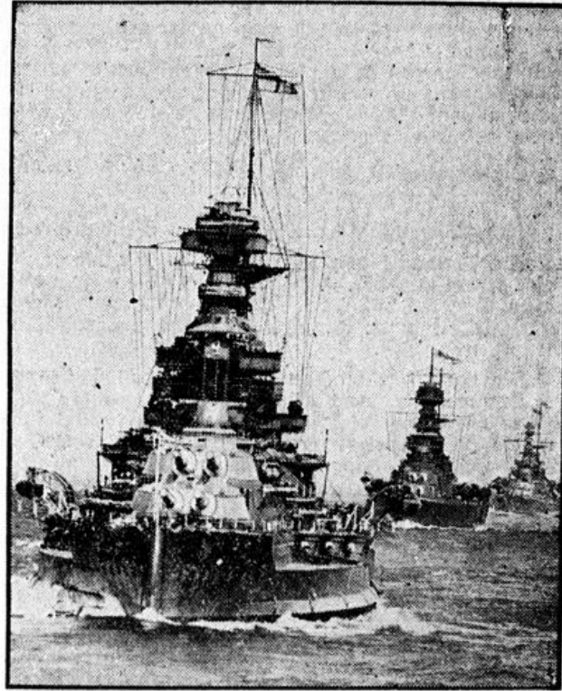
Weltbild (M).
