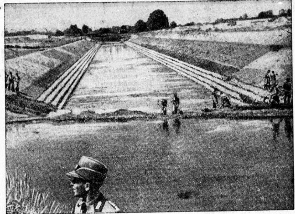
Regulierung der Ems durch den Arbeitsdienst Emsdurchstich bei Gimble in Westfalen. Der neue Flußlauf ist fertiggestellt und kurz vor dem Durchstich. Im Vordergrund der letzte Erd-damm, der die Ems noch vor dem Einströmen hindert. Durch die Regulierung werden die Ursachen der Stauungen beseitigt, die im Frühjahr oft Hochwasserständen brachten.
