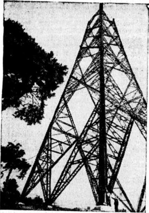
Das riesige Skelett des neuen Senders Tegel. Die moderne Technik verwendet das leichtere Holz an Stelle von Stahl.
