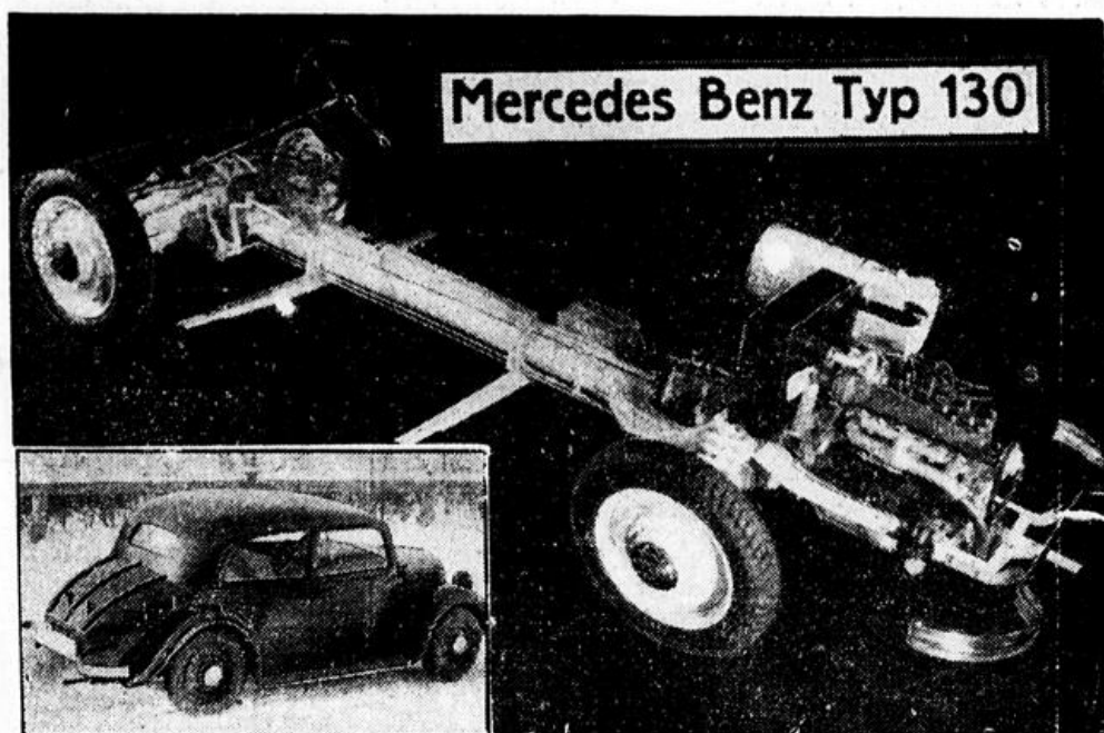
Mercedes Benz Typ 130 Revolution im Autobau. Das Chassis des Mercedes-Benz-Wagens Typ 130, bei dem der Motor hinten angebracht ist. Das rahmenlose Fahrgestell weist Schwingachsen auf. Unten links: Einer der schmucken Wagen des neuartigen Typs, der jetzt in Serienfabrikation als Volkswagen hergestellt wird. Die Heck-Motor-Konstruktion erspart die schwerwiegenden Motorübertragungsorgane von dem früheren Bug-Motor zu den Hinterrädern. Durch die Gewichtserparnis wird eine beträchtliche Schnelligkeitssteigerung erzielt.
