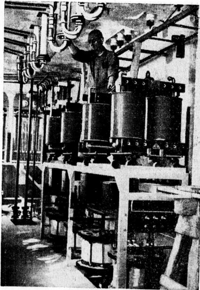
Geheimnisvolle Wunderwerke der Technik machen erst die Sendung möglich. Heiztransformatoren für die Großleistungsrohren.
