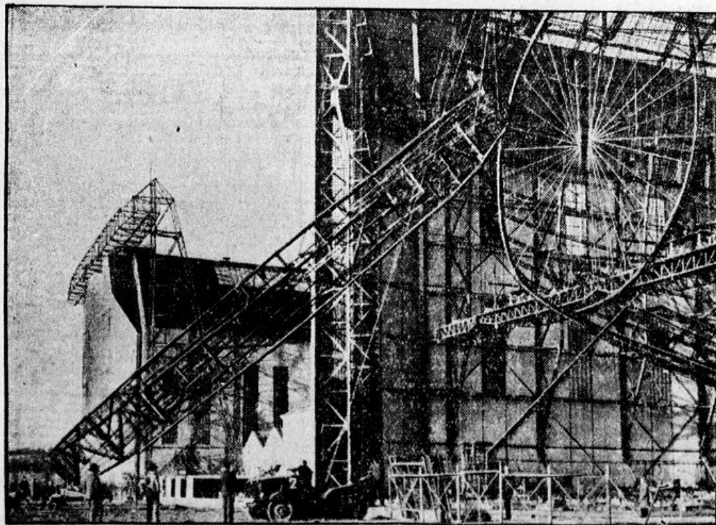
Blick in die neue Montagehalle bei Friedrichshafen, in der jetzt das deutsche Verkehrsflugschiff „Z 129“ gebaut wird. Unser Bild zeigt das Gerüst eines der letzten Bauringe.
