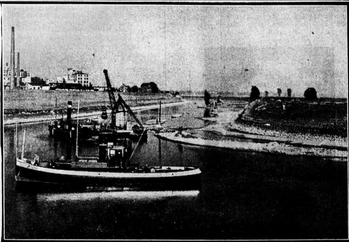
Der Stand der Hafen-Erweiterungsarbeiten an der Mündung.
