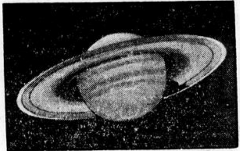
Der Ringplanet Saturn bei starker Vergrößerung.
