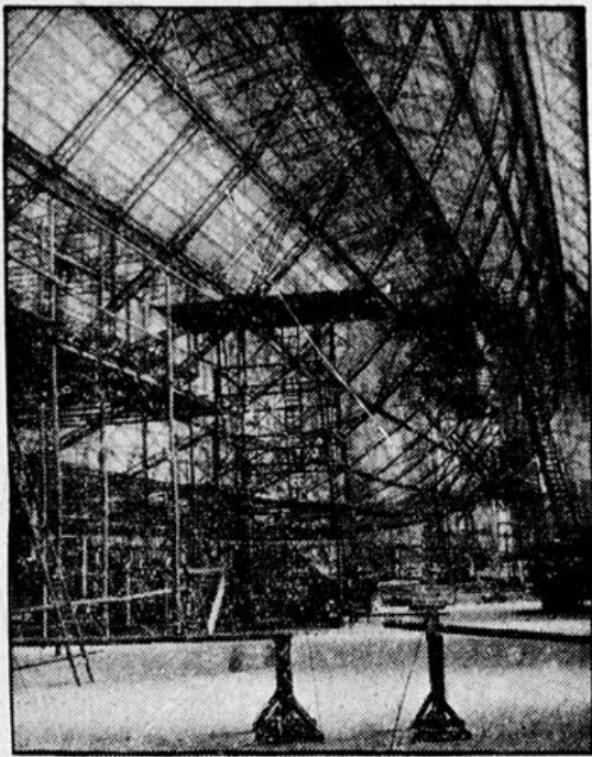
Das Gerüst des neuen deutschen Riesenluftschiffes „L Z 129“, das jetzt in Friedrichshafen seiner Vollendung entgegengeht.
