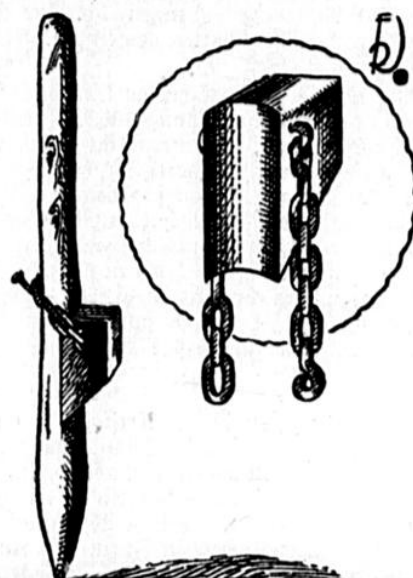
VORRICHTUNG ZUM RICHTIGEN SETZEN VON PFÄHLEN
