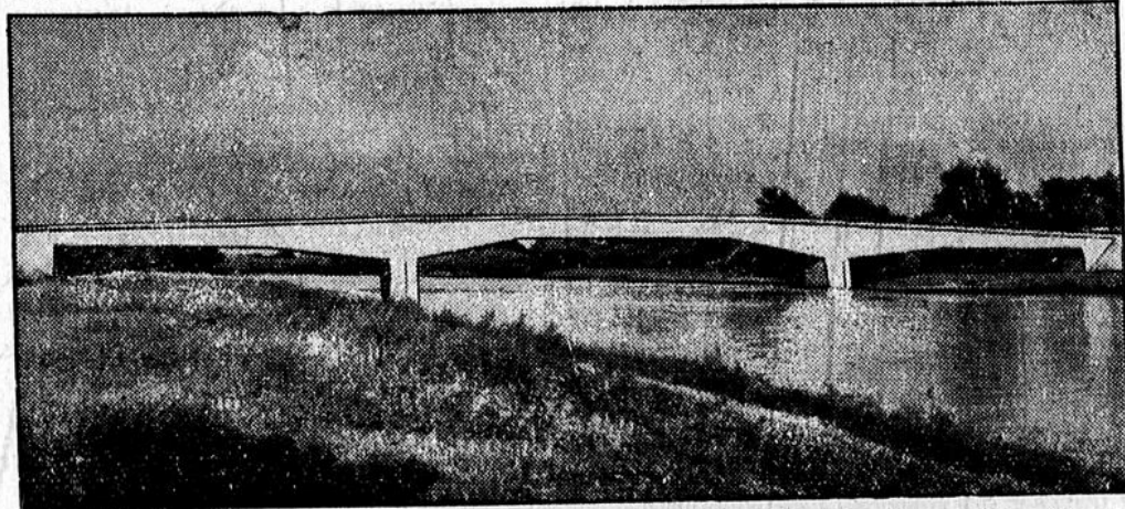
Die größte Eisenbeton-Valkenbrücke der Welt über die bayerische Donau Die neue Donaubrücke in Großmehring bei Ingolstadt, die größte Eisenbeton-Valkenbrücke der Welt, wird am 31. August ihrer Bestimmung übergeben.
