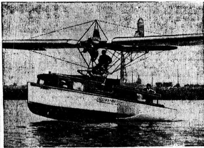
Segelflugzeugstart vom Motorboot.
