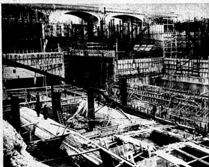
Gewaltige Gerüste sind zum Bau der Schleuse bei Anderten nötig. — Rechts: Ein Brückenbogen am Unterhaupt der Schleuse bei Anderten wird eingeschalt
