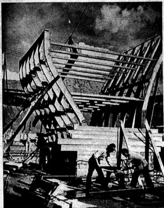
Bei der Verschalung eines Abfallschachtes für das Oberwasser am Oberhaupt der Schleuse bei Anderten (bei Hannover)
