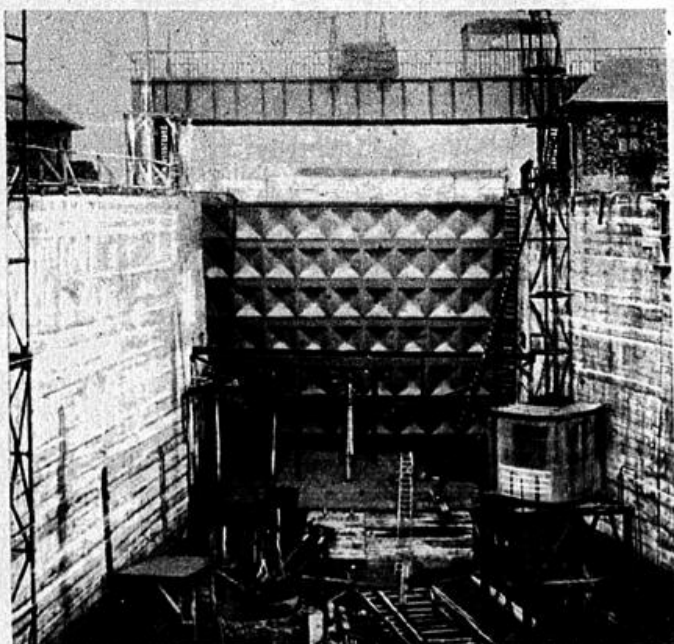
Die zweite Mündung des Rhein-Herne-Kanals in Duisburg; eines der drei 100-Tonnen-Schleusentore
