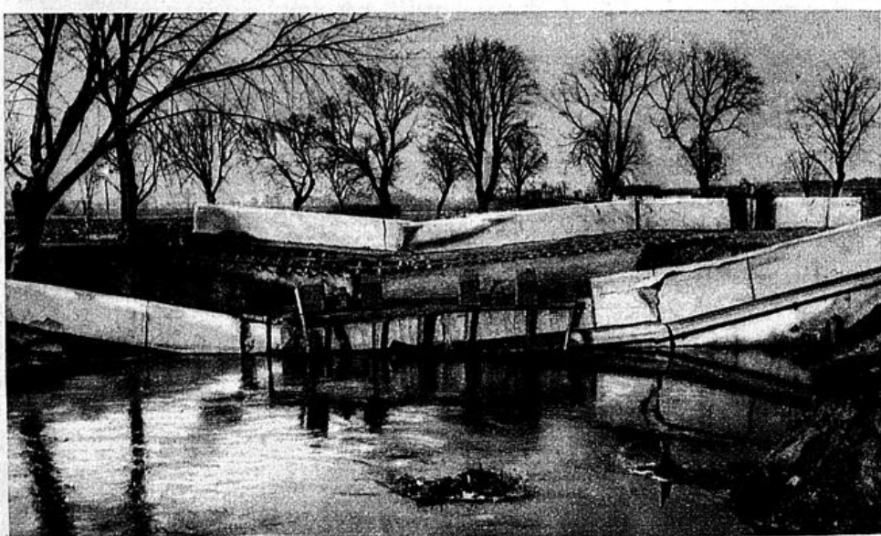
In der Nähe von Liebenwalde stürzte die 14 Meter lange Eisenbetonbrücke über die Havel im Zuge der Chaussee Liebenwalde-Niederbarnim ein. Die Betonpfeiler der Brücke waren von den stark angeschwollenen Wassermassen der Havel unterpült worden
