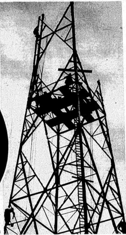
Vom Bau des Rhein-Ruhr-Senders, der auf der Hardt in Langenberg (Rhld.) errichtet wird und im Dezember in Betrieb genommen werden soll
