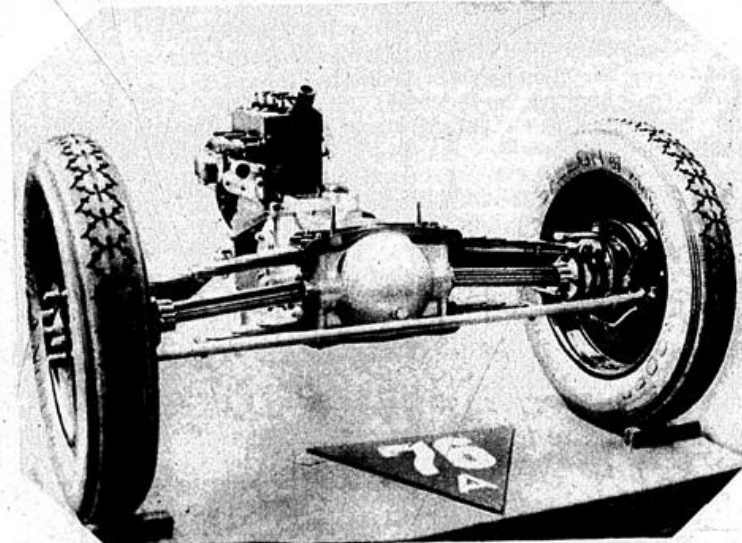
Die Vorderachse der neuesten „Boran-Wagen“, bei denen der Antrieb nicht mehr an der Hinter-, sondern an der Vorderachse erfolgt Atlantic
