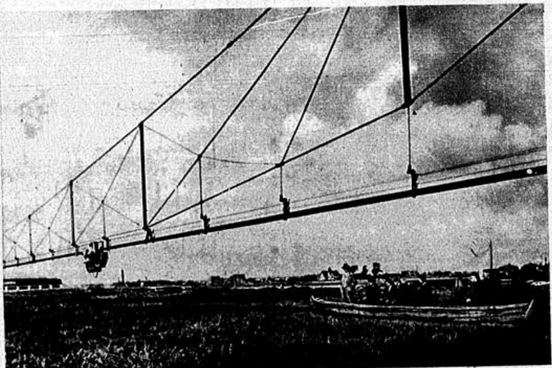
Der Erleichterung des Schiffsverkehrs auf den Binnenwasserstraßen soll eine neue Erfindung dienen, bei der eine in Längsrichtung des Kanals angelegte elektrische Schwebebahn das Schleppen von Rähnen und anderen Fahrzeugen übernimmt. — Praktische Versuche auf einer Probefstrecke Presse-Archiv
