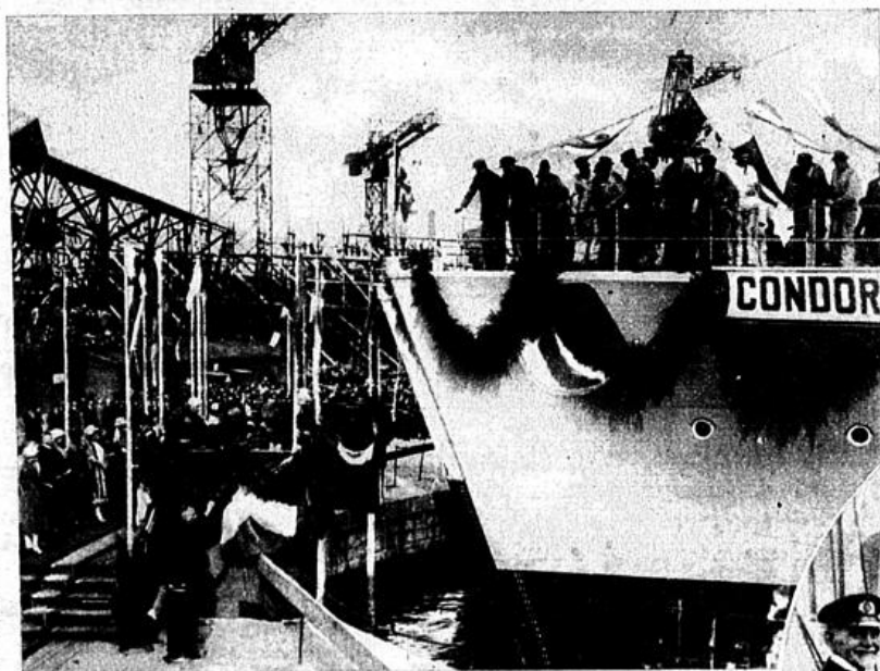
Bild oben: Vom Stapellauf der beiden neuen großen Torpedoboote der Reichs- marine „Condor“ und „Falke“ auf der Wilhelms- havener Marinewerft: Der „Condor“ nach der Taufe Sennede
