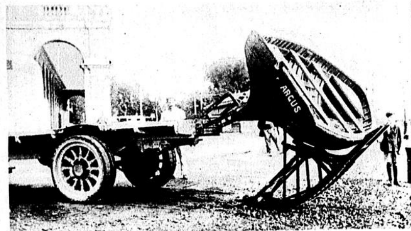
Eine einfache, aber höchst sinnreiche Vorrichtung, die das Auf- und Abladen von Waren mechanisiert Oben: Die erste Phase des Hebens, der Schlitten gleitet aufwärts; unten: Die Brücke des Schlittens in horizontaler Lage. Der ganze Vorgang vollzieht sich nach dem Befehl des Hebels
