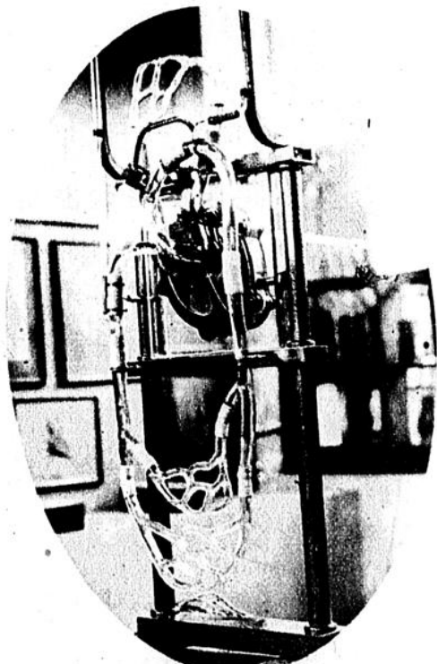
Eine einfache, aber höchst sinnreiche Vorrichtung, die das Auf- und Abladen von Waren mechanisiert Oben: Die erste Phase des Hebens, der Schlitten gleitet aufwärts; unten: Die Brücke des Schlittens in horizontaler Lage. Der ganze Vorgang vollzieht sich nach dem Befehl des Hebels
