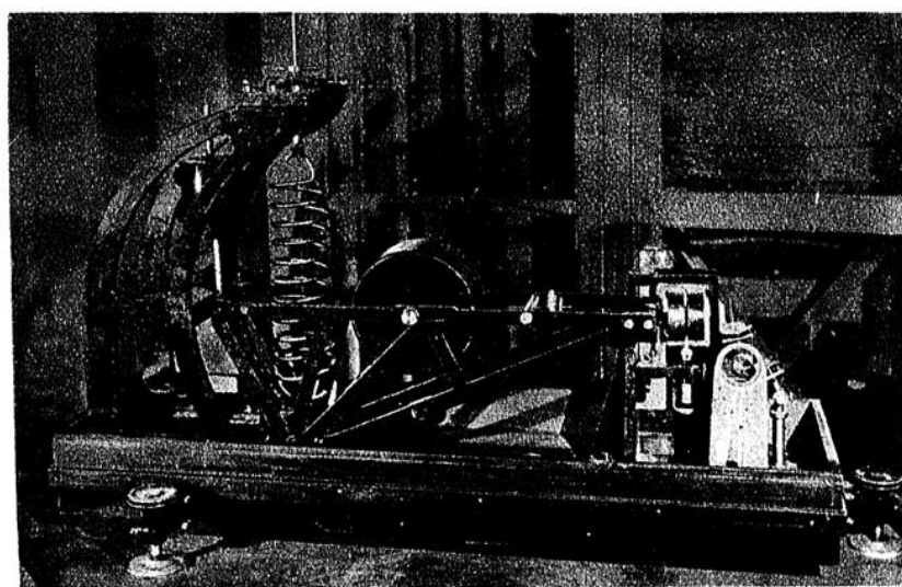
Seismograph nach Jallin für die Vertikalkomponente der Bodenbewegung mit magnetischer Dämpfung für photographische Registrierung mit drei Spiegeln
