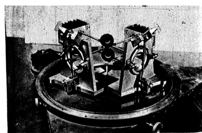
Horizontal-Pendelapparat mit Luftdämpfung zur photographischen Aufzeichnung der Nord-Süd-Ost-West-Komponente der horizontalen Bodenbewegung
