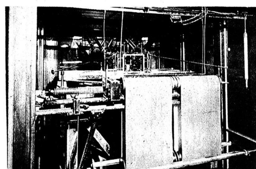
Horizontal-Seismograph zur Aufzeichnung der Nord-Süd- und Ost-West-Komponente der horizontalen Bodenbewegung für mechanische Registrierung
