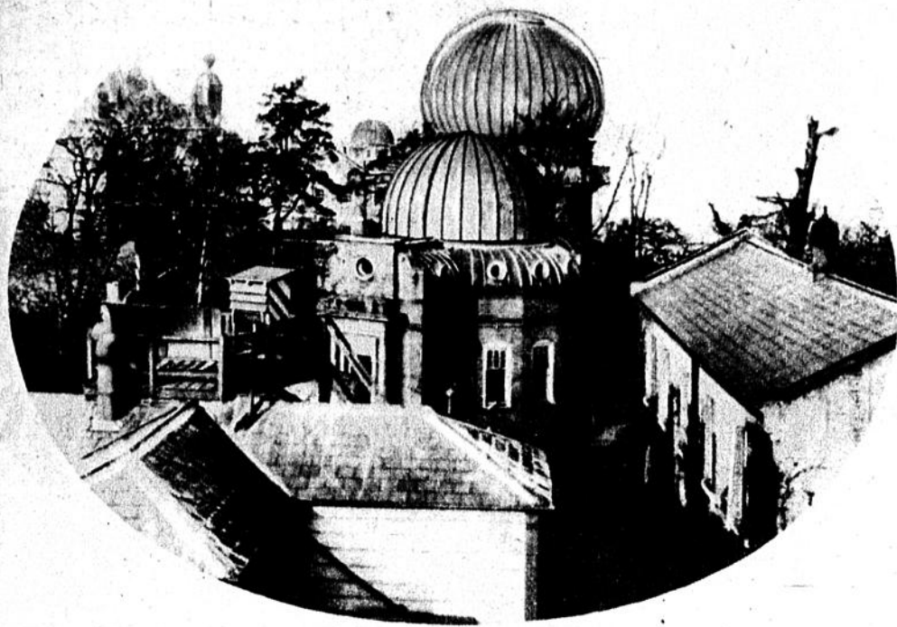
Die bekannte englische Sternwarte in Greenwich (England) kann auf ein 250jähriges Bestehen zurückblicken
