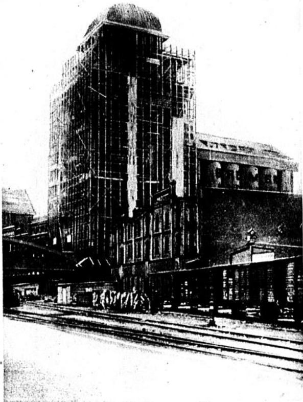
Das höchste industrielle Hochhaus Europas, das Geschäftshaus der Bremer Roland-Mühle A.-G. im Rohbau
