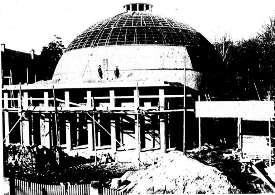
Das Zeiss-Planetarium in Jena vor der Vollendung
